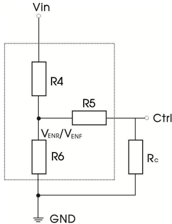
可调输入启动 (欠压) 电压的使用电路(虚线框为产品内部)
