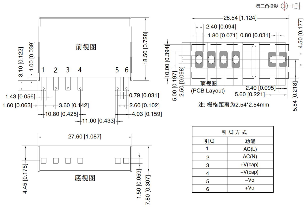
LS05-23BxxDR3 系列外观尺寸图
