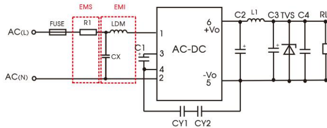
应用电路 2
