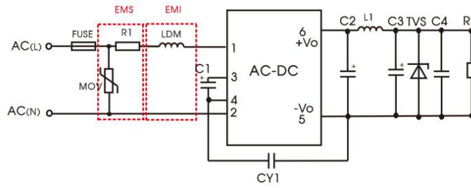
应用电路 4
