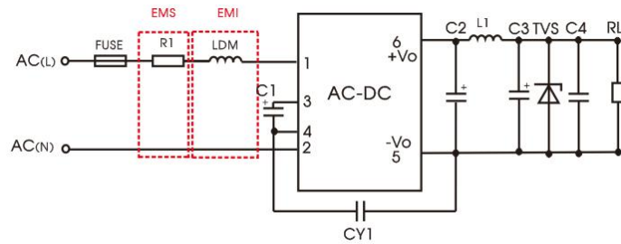
应用电路 1
