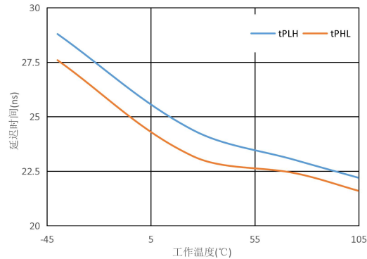
图7. 驱动器延时 vs. 工作温度
