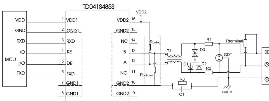
图 14 端口保护推荐电路
