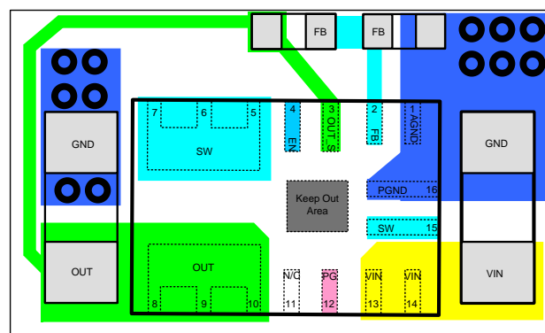
Top Layer
