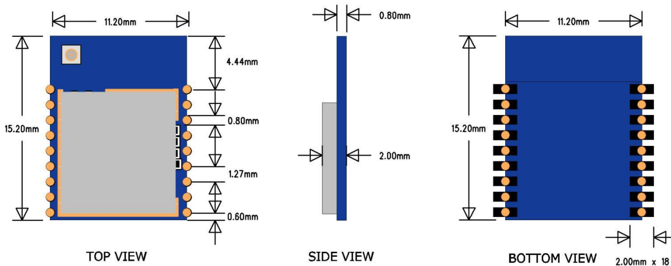
图2 模块尺寸图
