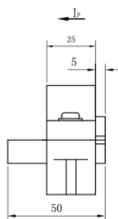
左视图
