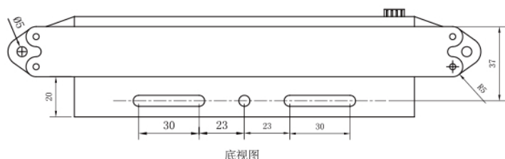
底视图
