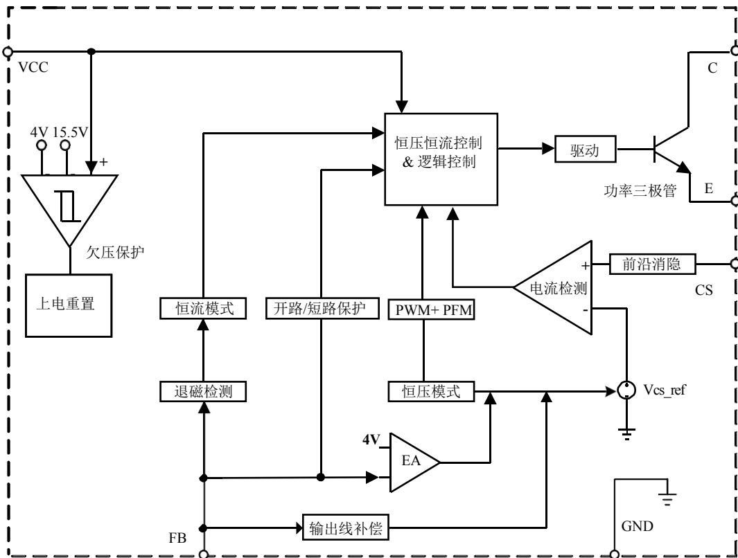
图 3 ICW3773CA/B 内部框图
