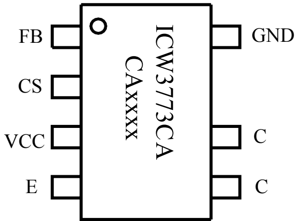
图 2 ICW3773CA管脚封装图
