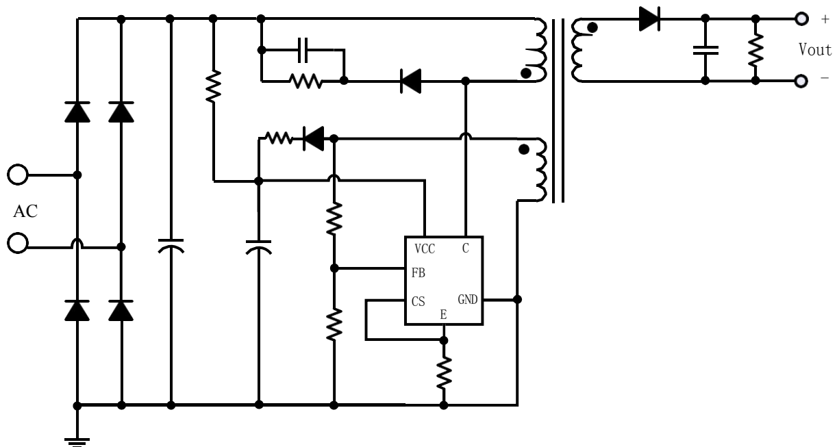
图 1 ICW3773CA/B 典型应用图
