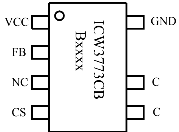
图 3 ICW3773CB管脚封装图
