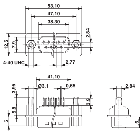
尺寸图
