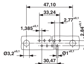
钻孔图
