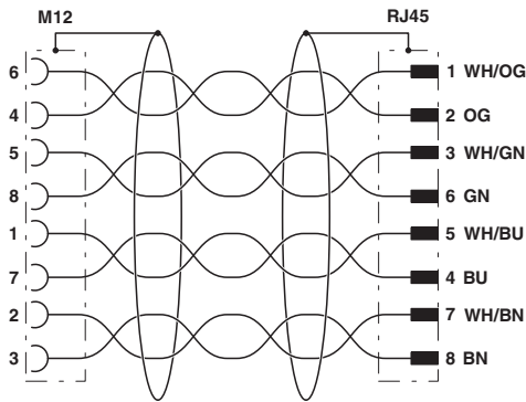
电路图
