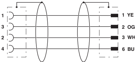
电路图
