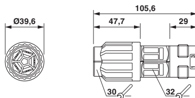
尺寸图
