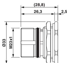
尺寸图
