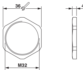
尺寸图
