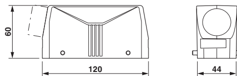
尺寸图
