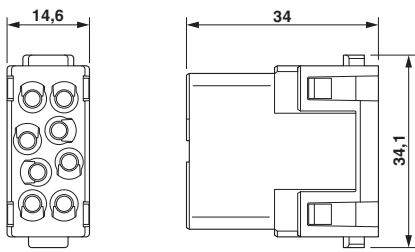
尺寸图
