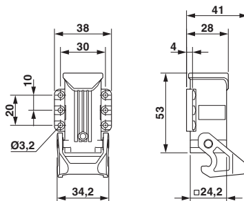
尺寸图
