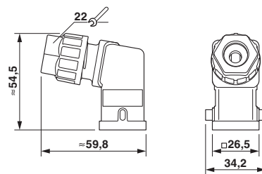
尺寸图
