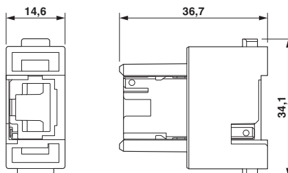
尺寸图
