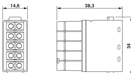
尺寸图
