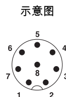
M8针式连接器引脚分配, 8芯, 插头侧视图
