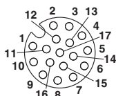
M12针脚分配, 17芯, 插座侧视图
