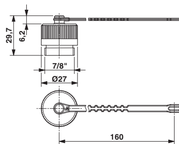
尺寸图
