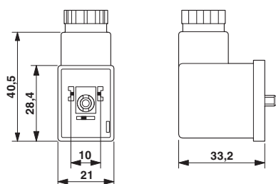
尺寸图
