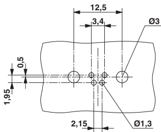
钻孔图
