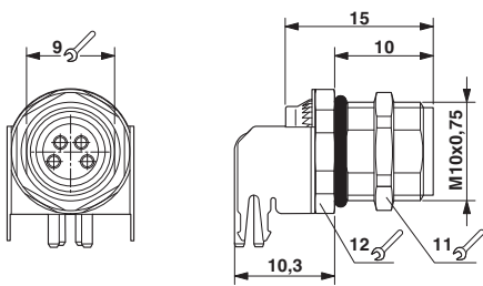
尺寸图
