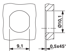
尺寸图
