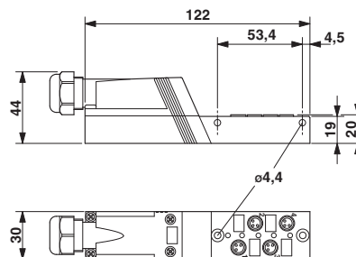
尺寸图
