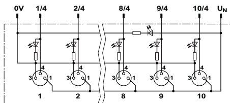
电路图
