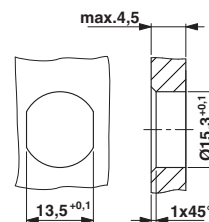
尺寸图
