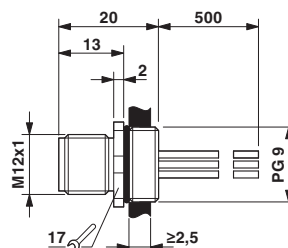
尺寸图
