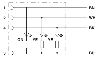
电路图
