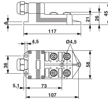
尺寸图
