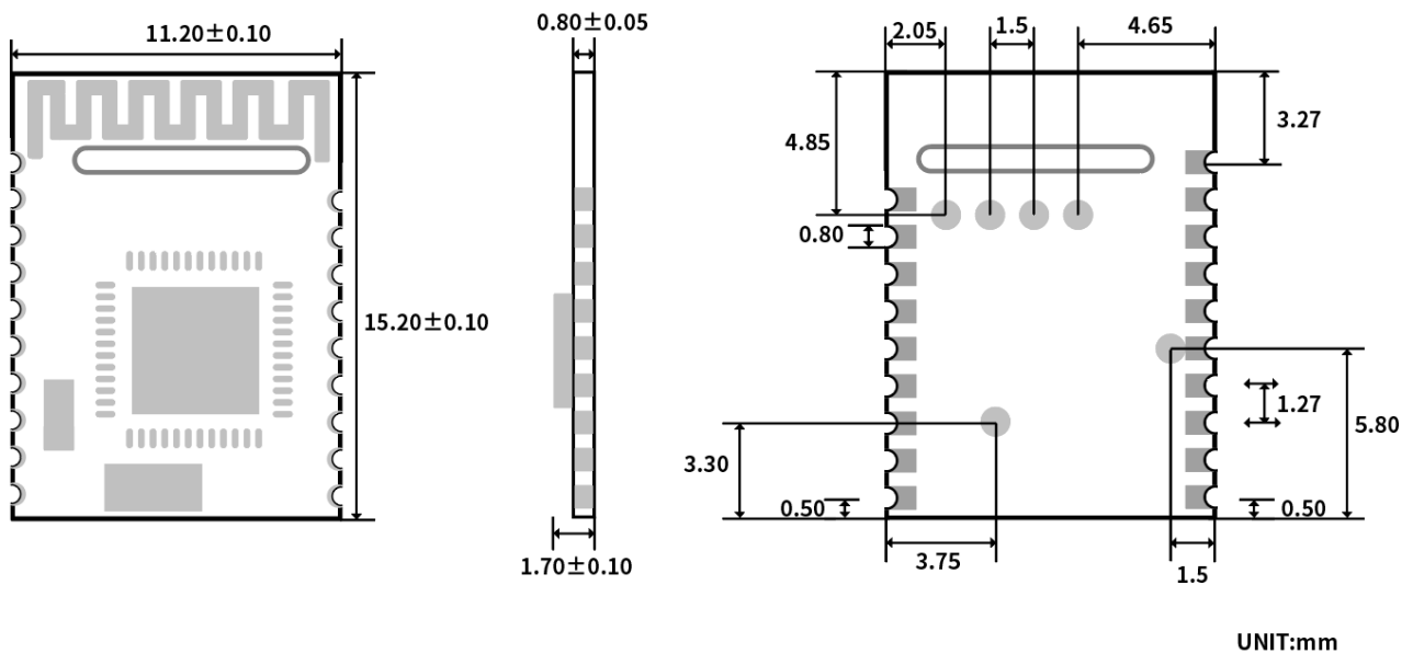
图 2. RF-BM-ND08C 尺寸图
