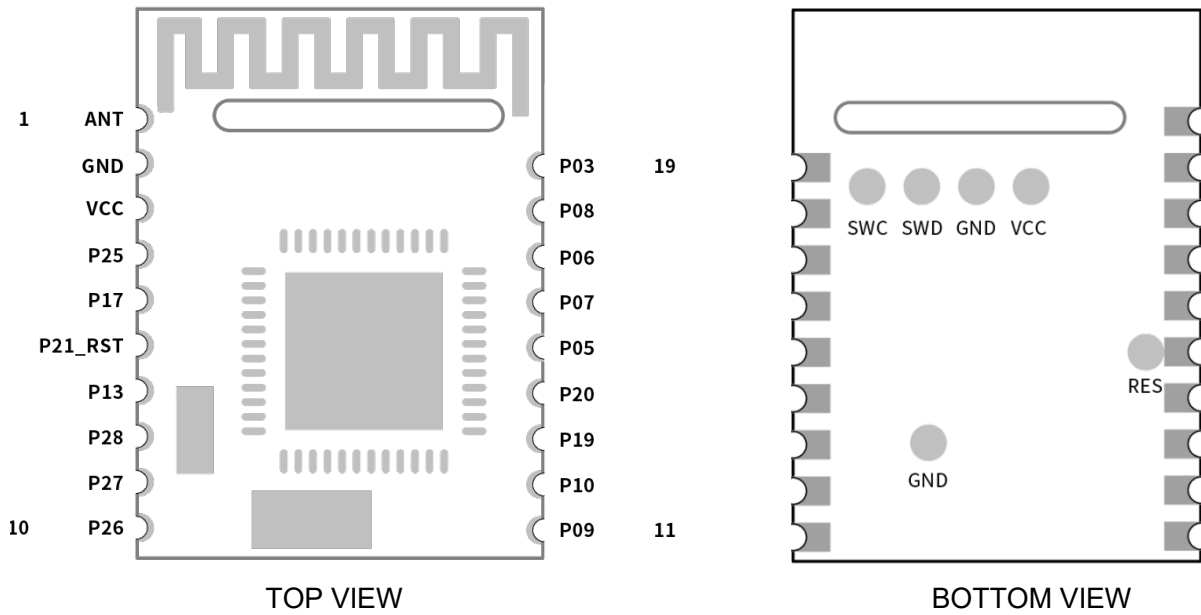
图 3. RF-BM-ND08C 引脚图
