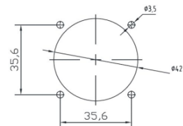
客户面板开孔尺寸图
