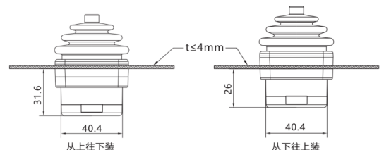
机械安装图
