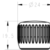
K2上端尺寸图
