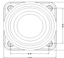
俯视图
