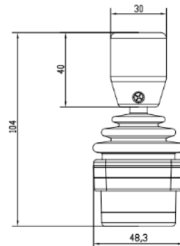
正视图
