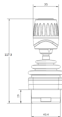
正视图
