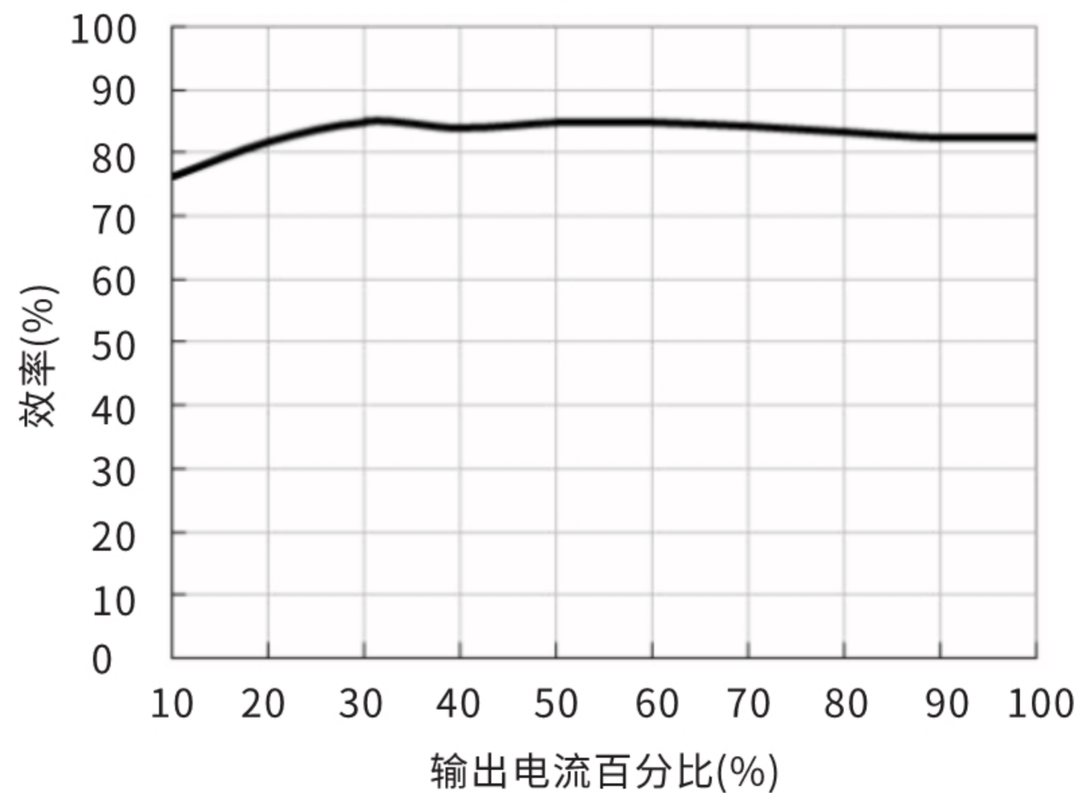
效率Vs输出负载(Vin=5V)
