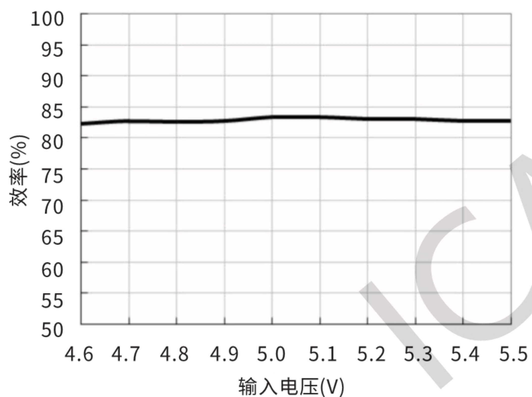
效率Vs输入电压(满载)
