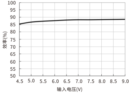
效率Vs输入电压(满载) VRB0524ZP-6WR3
