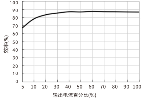
效率Vs输出负载(Vin=5V) VRB0524ZP-6WR3
