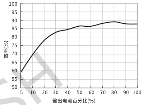
效率Vs输出负载(Vin=48V) VRB4824ZP-6WR3
