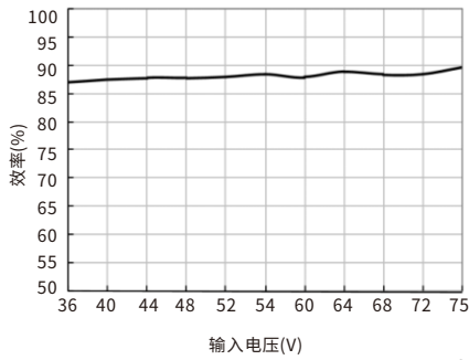
效率Vs输入电压(满载) VRB4824ZP-6WR3
